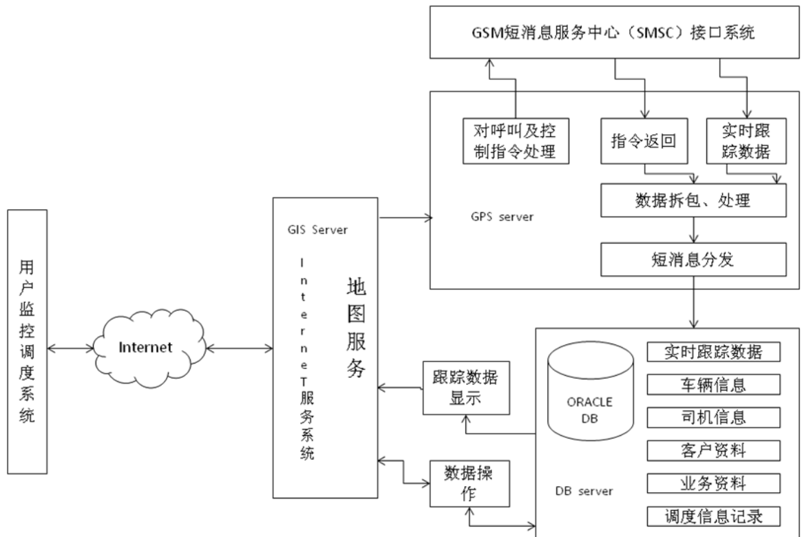
图7 车辆监控系统业务流程图
